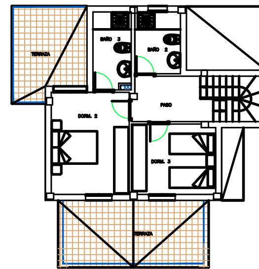
PLANTA PRIMERA
