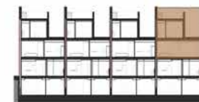
Sección Bloque 3
