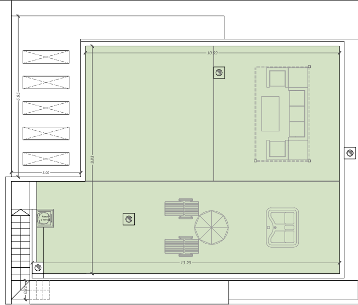
PLANTA CUBIERTA-SOLARIUM
